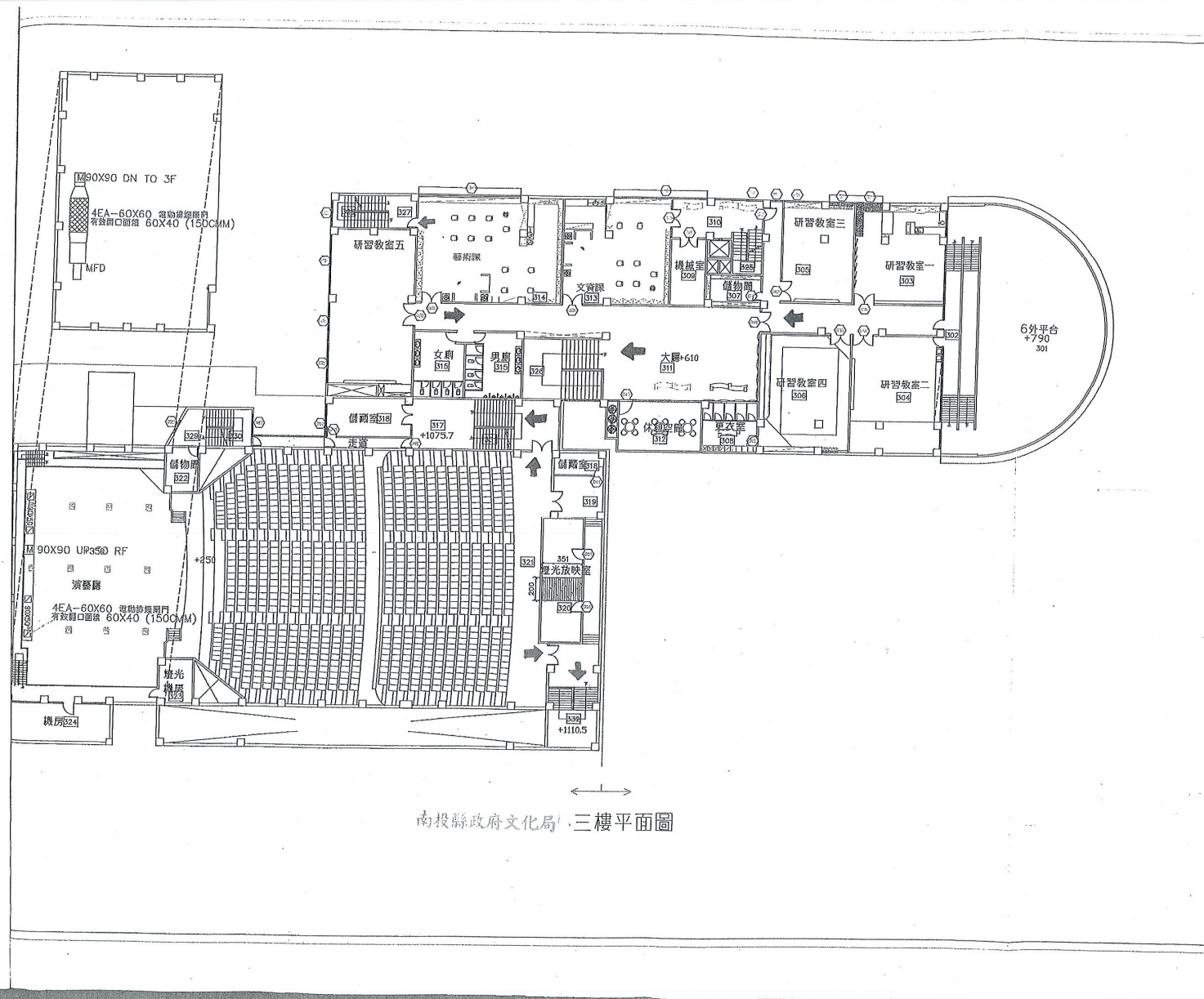
圖 5. 南投縣政府文化局 3 樓平面圖
